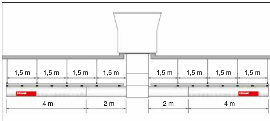
TopVent® / TopVent® 9-es méret 2-oldali
