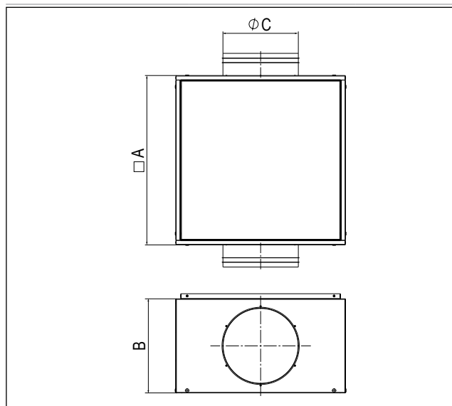
Kép: TopVent készülék légalosztó dobozzal
