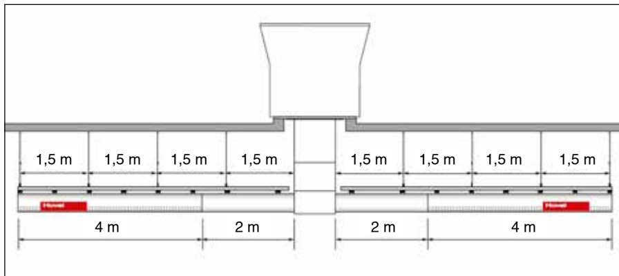
TopVent® / TopVent® 6-os méret 2-oldali
