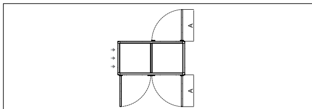
Kép: Minimális távolságok a P hőszivattyúhoz (mm-ben)
