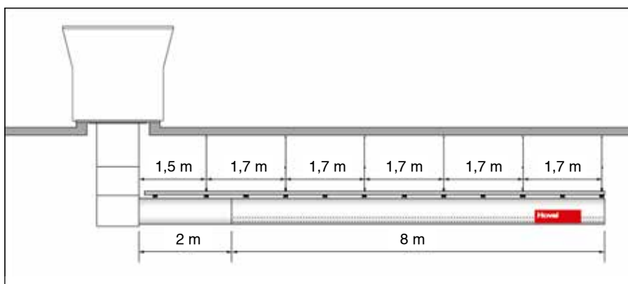
TopVent® / TopVent® 6-os méret 1-oldali
