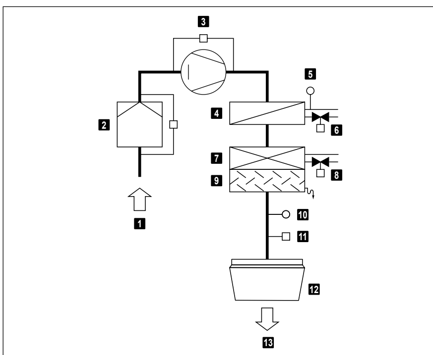
Kép: TopVent® CHC működési vázlata
