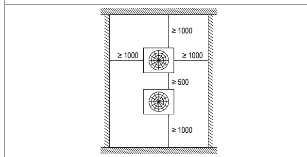
Kép: Minimális távolságok a Q hőszivattyúhoz (mm-ben)
