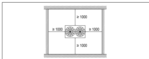
Kép: Minimális távolságok a P hőszivattyúhoz (mm-ben)
