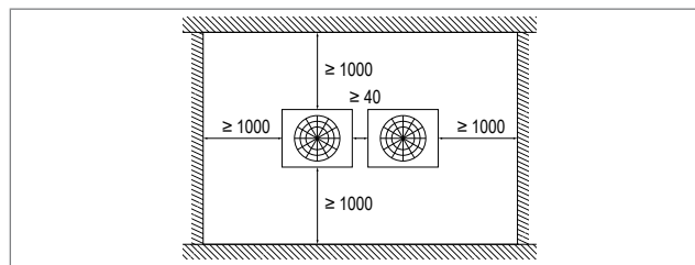
Kép: Minimális távolságok a P hőszivattyúhoz (mm-ben)
