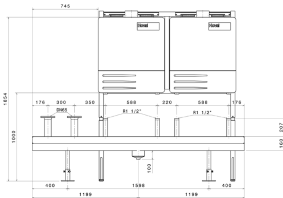
Előlnézet
