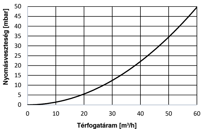
Hoval UltraGas® 2 (620-700)
