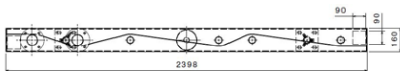
Felülnézet
