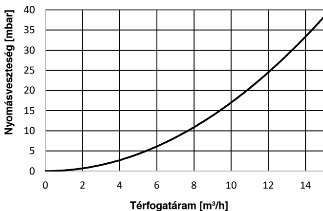
Hoval UltraGas® 2 (125, 150)
