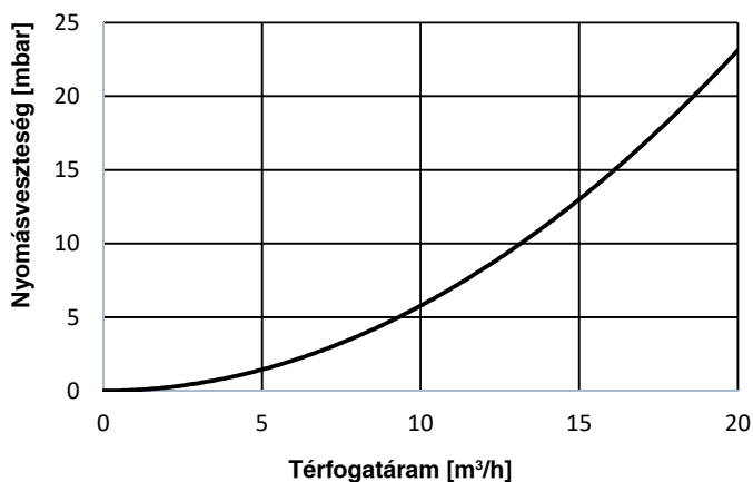
Hoval UltraGas® 2 (190, 230)
