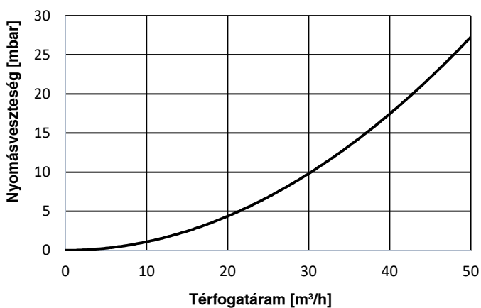
Hoval UltraGas® 2 (300-500)
