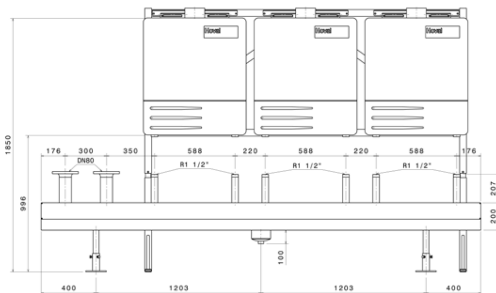
Előlnézet
