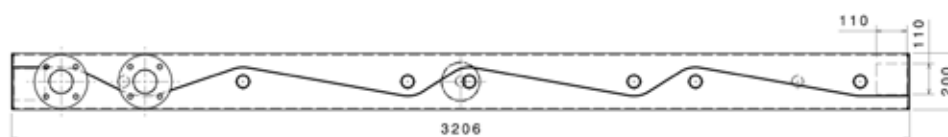
Felülnézet
