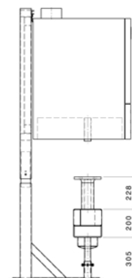
Bal nézet
