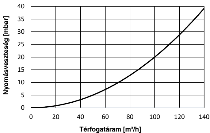
Hoval UltraGas® 2 (1300, 1550)
